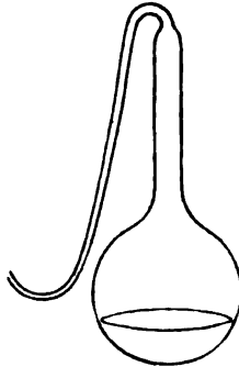
PASTEUR'S FLASK.
